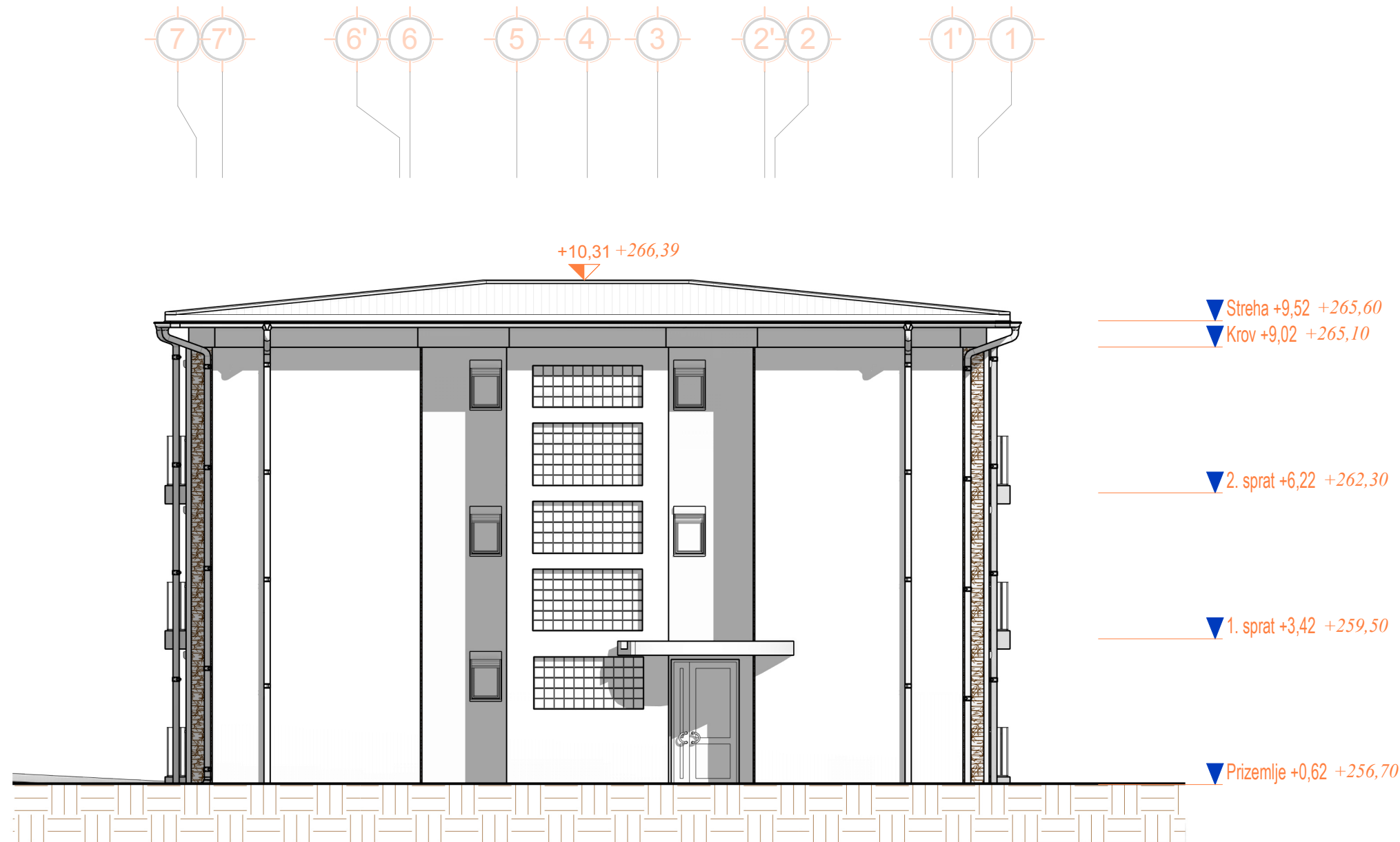
1 Severoistočni izgled- 1 : 100
