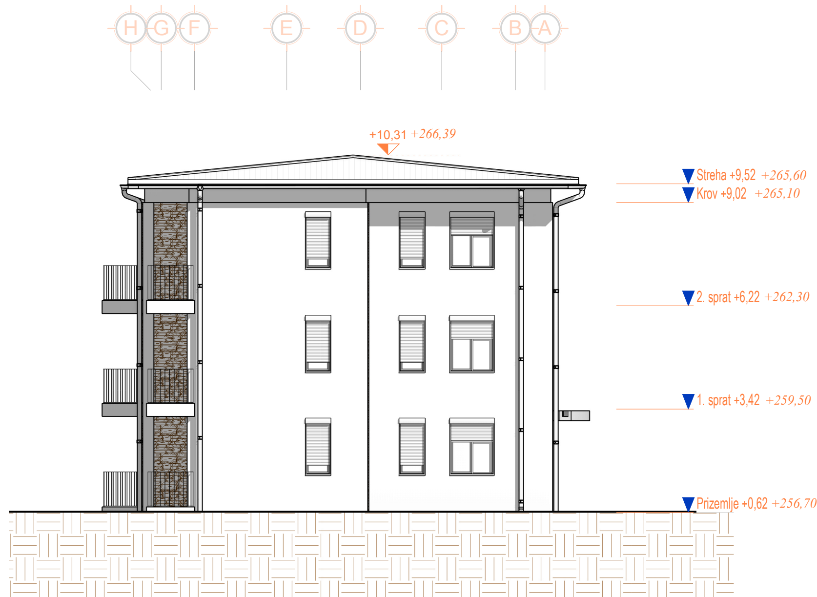
2 Jugoistočni izgled 1 : 100
